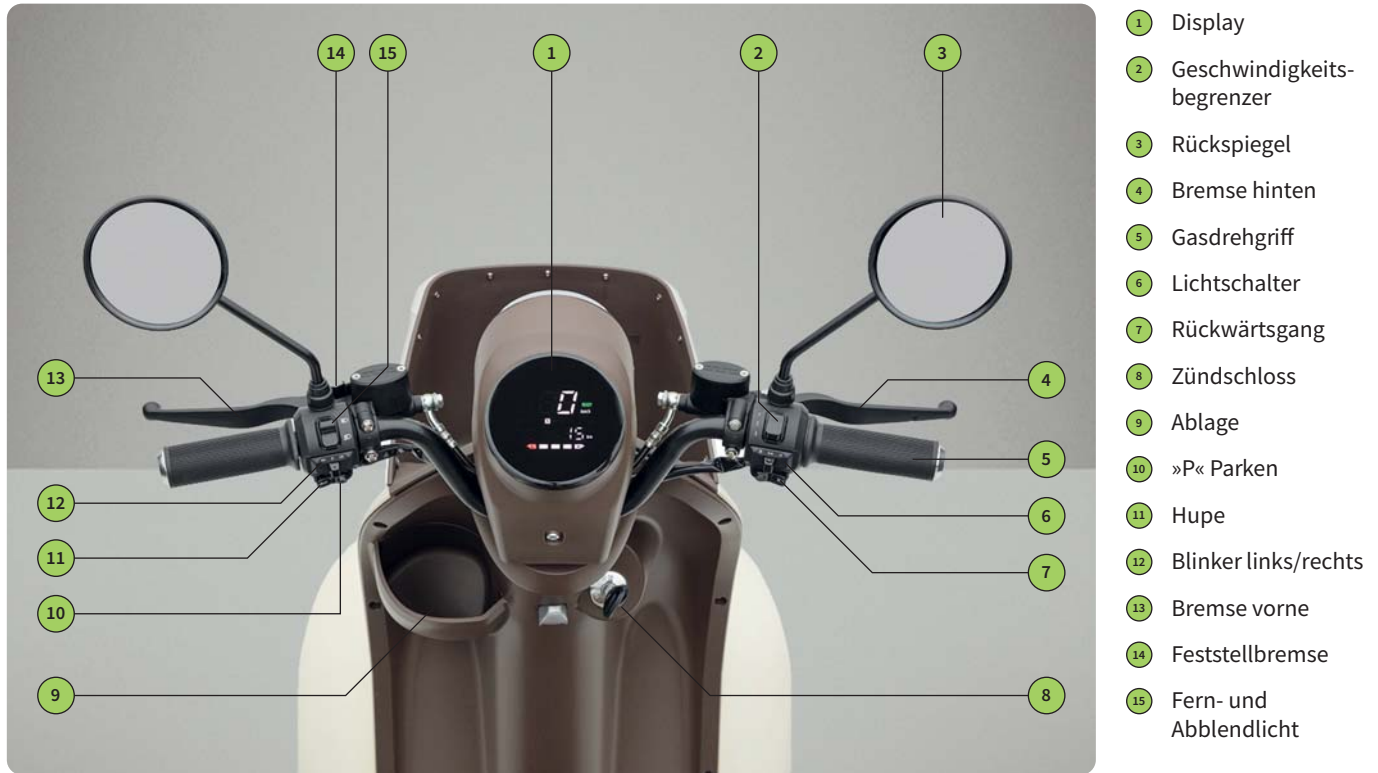
Abb. 1.6 Bedienelemente des Fahrzeugs
