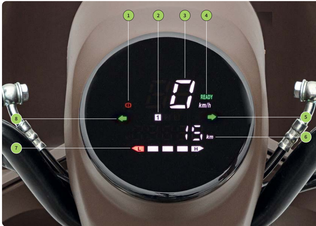
Abb. 1.7 Anzeige und Display des Fahrzeugs
